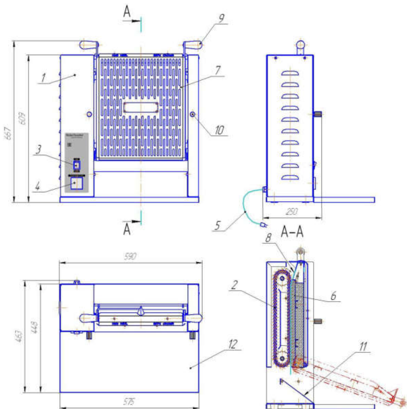
Рис. 1 Тостер.
